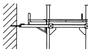
Diagonalstag som långkruss. Påbörjas alltid i ytterråmen.
