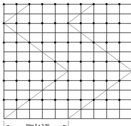
Diagonalstag som långkruss. Påbörjas alltid i ytterråmen.
