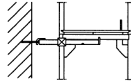
V-förankring
